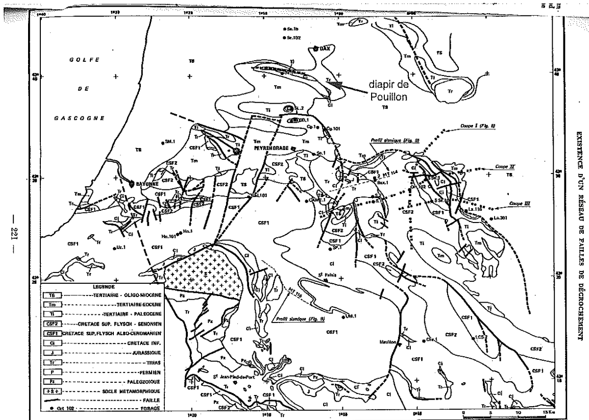
FIGURE 2 (Zolnai, 1975) Carte géologique. Geologic map.
